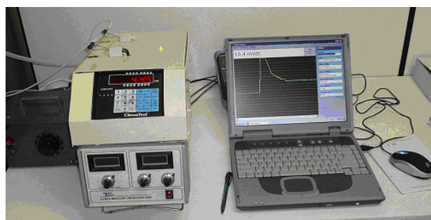
Figura 1. Sistema analítico de dessorção e detecção de Hg construído sobre detector Tekran 2500.
